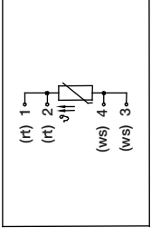
1 x Pt100 / 4-Leiter / wire / fils
